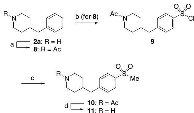
Scheme 3. Reagents: (a) \text{Ac}_2\text{O} ; (b) \text{ClSO}_3\text{H} , DCM; (c) \text{Na}_2\text{SO}_3 , \text{NaHCO}_3 , \text{H}_2\text{O} , then \text{ClCH}_2\text{CO}_2\text{H} , aq NaOH; (d) concd HCl, then aq NaOH.
