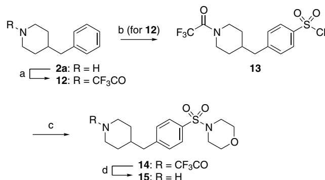
Scheme 4. Reagents: (a) TFAA; (b) \text{ClSO}_3\text{H} , DCM; (c) morpholine, \text{Et}_3\text{N} , THF; (d) \text{K}_2\text{CO}_3 , \text{H}_2\text{O} , MeOH.
